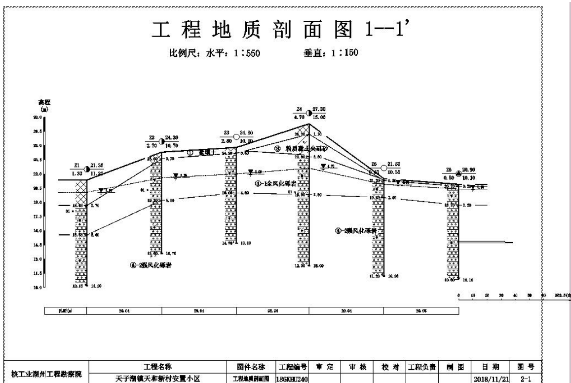
图 3-5 部分点位工程地质剖面图
